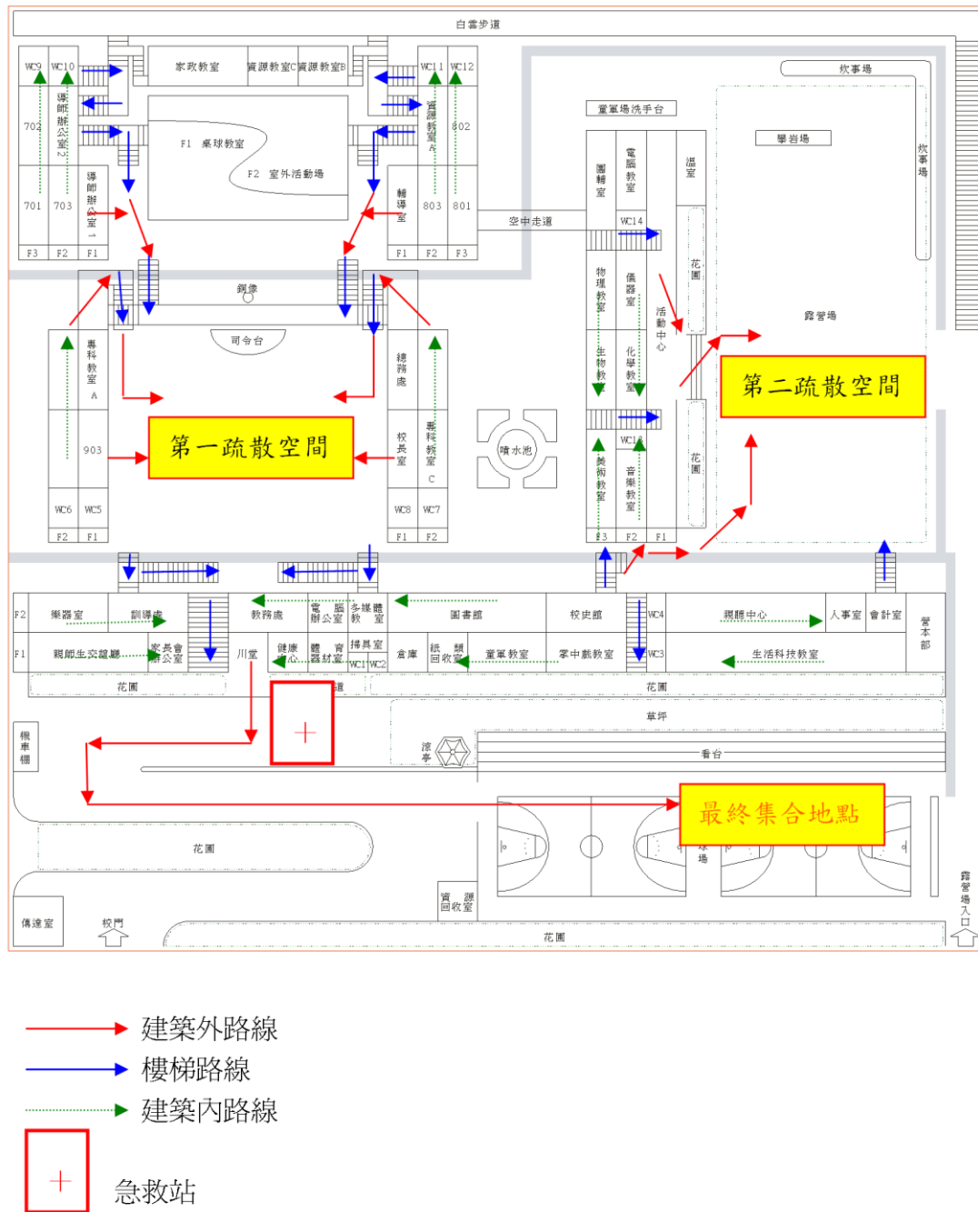
圖 8-2-3、避難逃生路線圖
