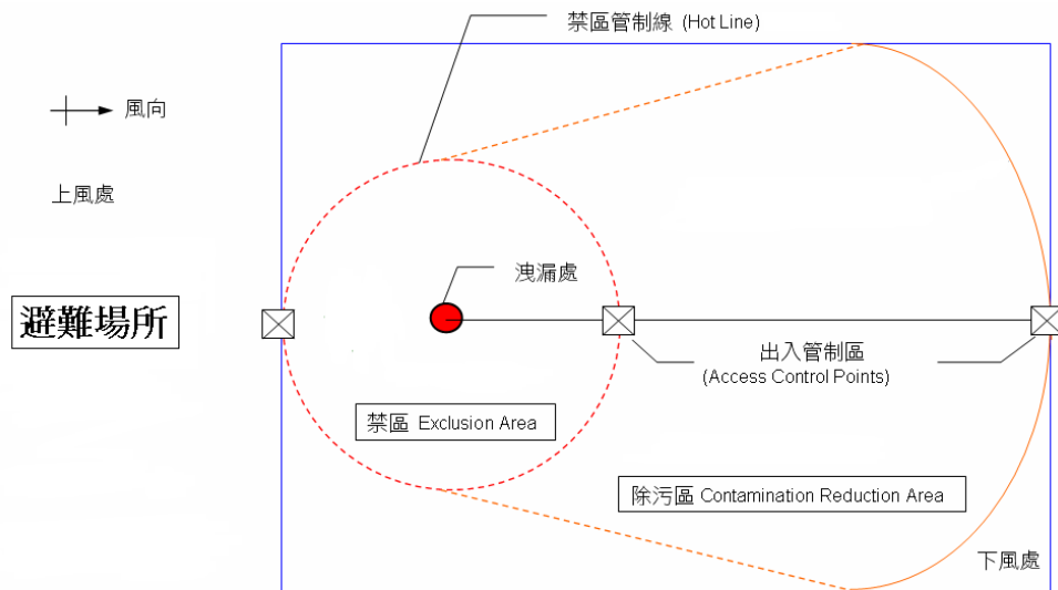
圖 12-6-1、避難場所區域劃分示意圖
