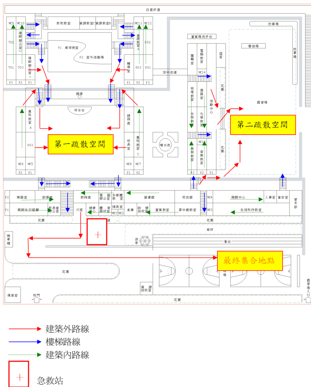
臺北市立格致國民中學地震災害學生緊急疏散路線示意圖
