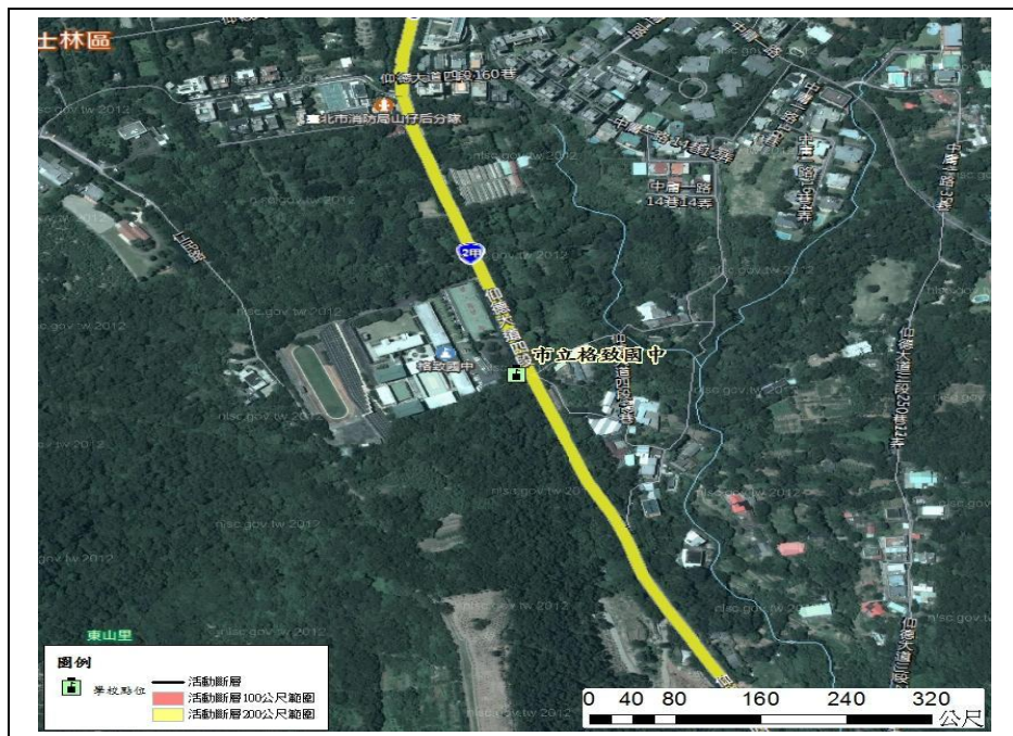
2-2-1、活動斷層圖
